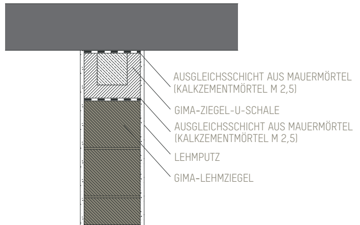
TRAGENDE INNENWAND AN „HOLZDECKE“
